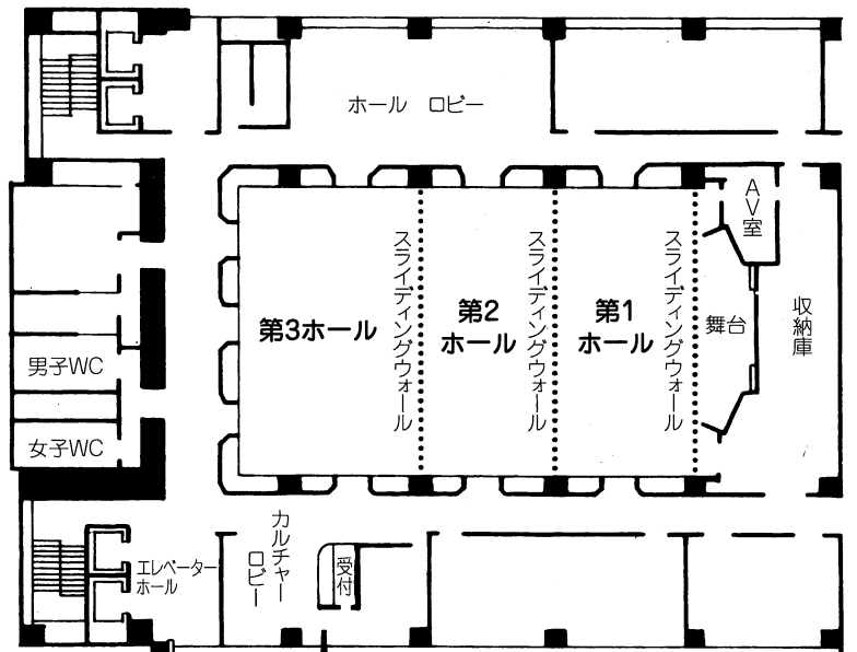
京都新聞文化ホール平面図
